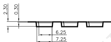
SECTION A-A SCALE 1:1
